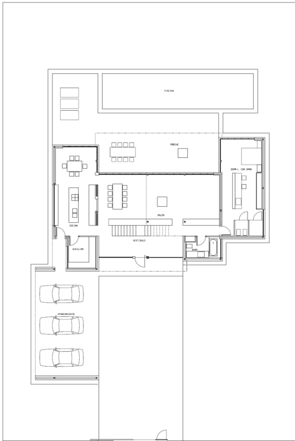
4D-dúplex planta baja
