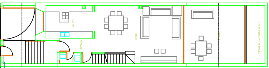
3D-1 en hilera Planta baja
