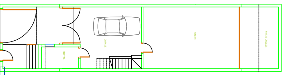
3D-2 en hilera Semisótano
