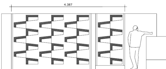
Cerramiento de parcela Solución 2 Exterior
